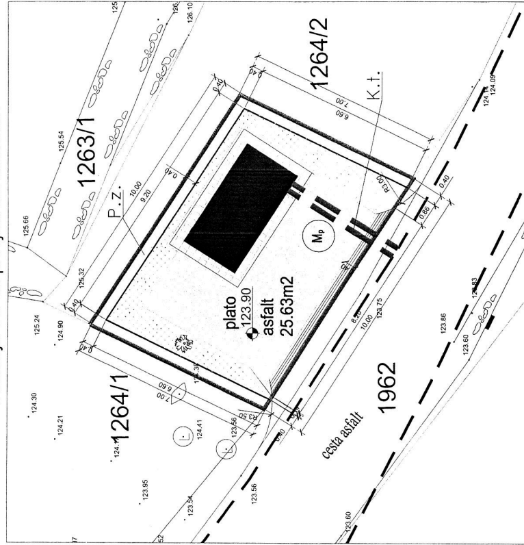
Situacija TS sa priključnim kabelom
