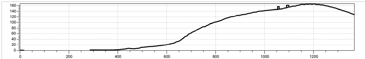
Grafički prikaz 37: Položajna točka ljetnikovac Sorkočević sa presjekom terena – varijanta 2
