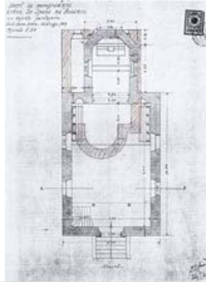
Projekt rekonstrukcije crkve sv. Spasa iz 1914. g.
