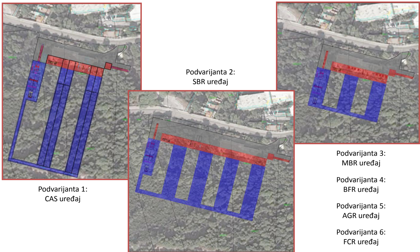
Slika 2.3: Situacijski prikaz smještanja UPOV-a na osnovi različitih podvarijanti biološkog postupka pročišćavanja.
